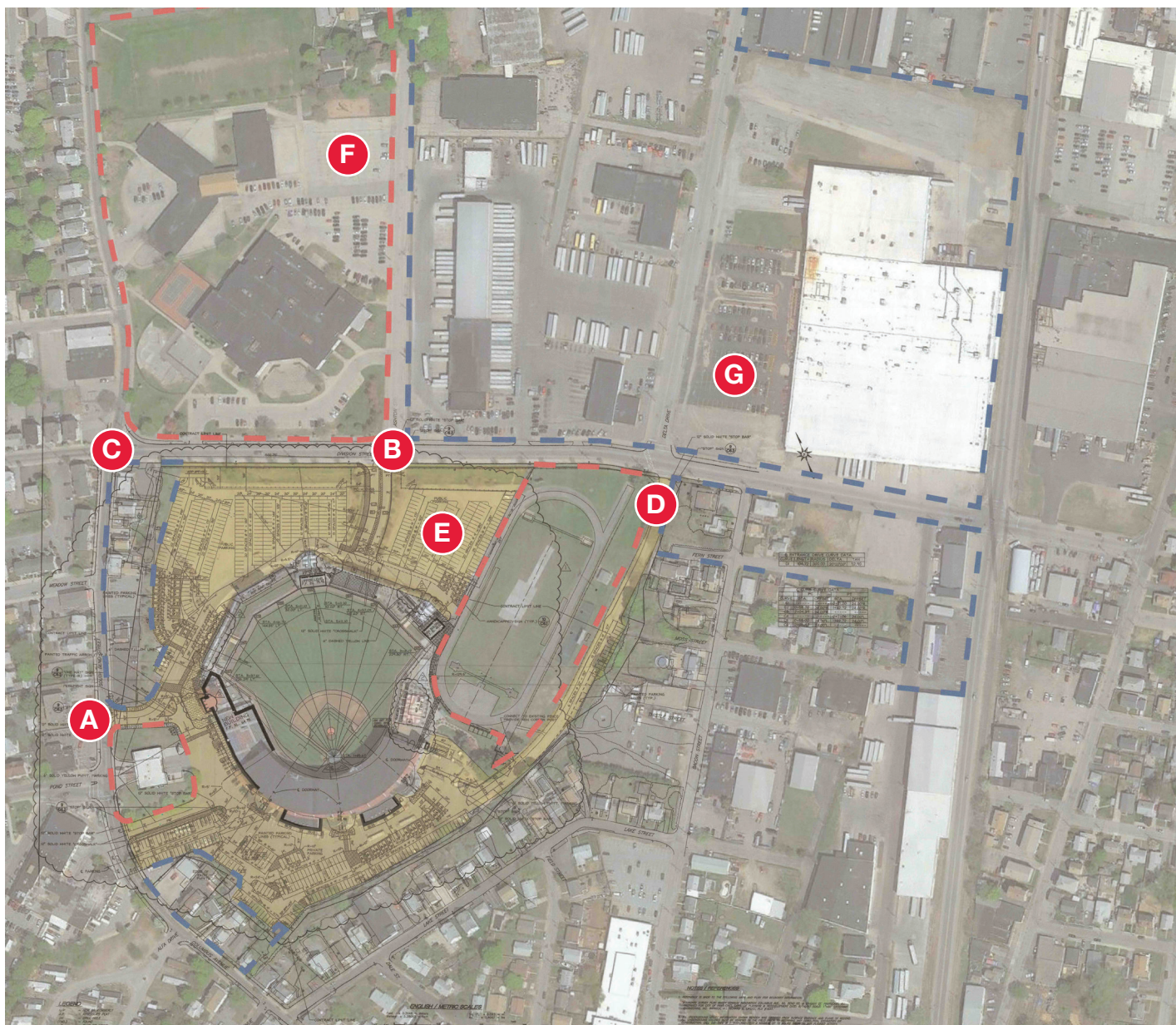
Fig. 015. Site Plan
